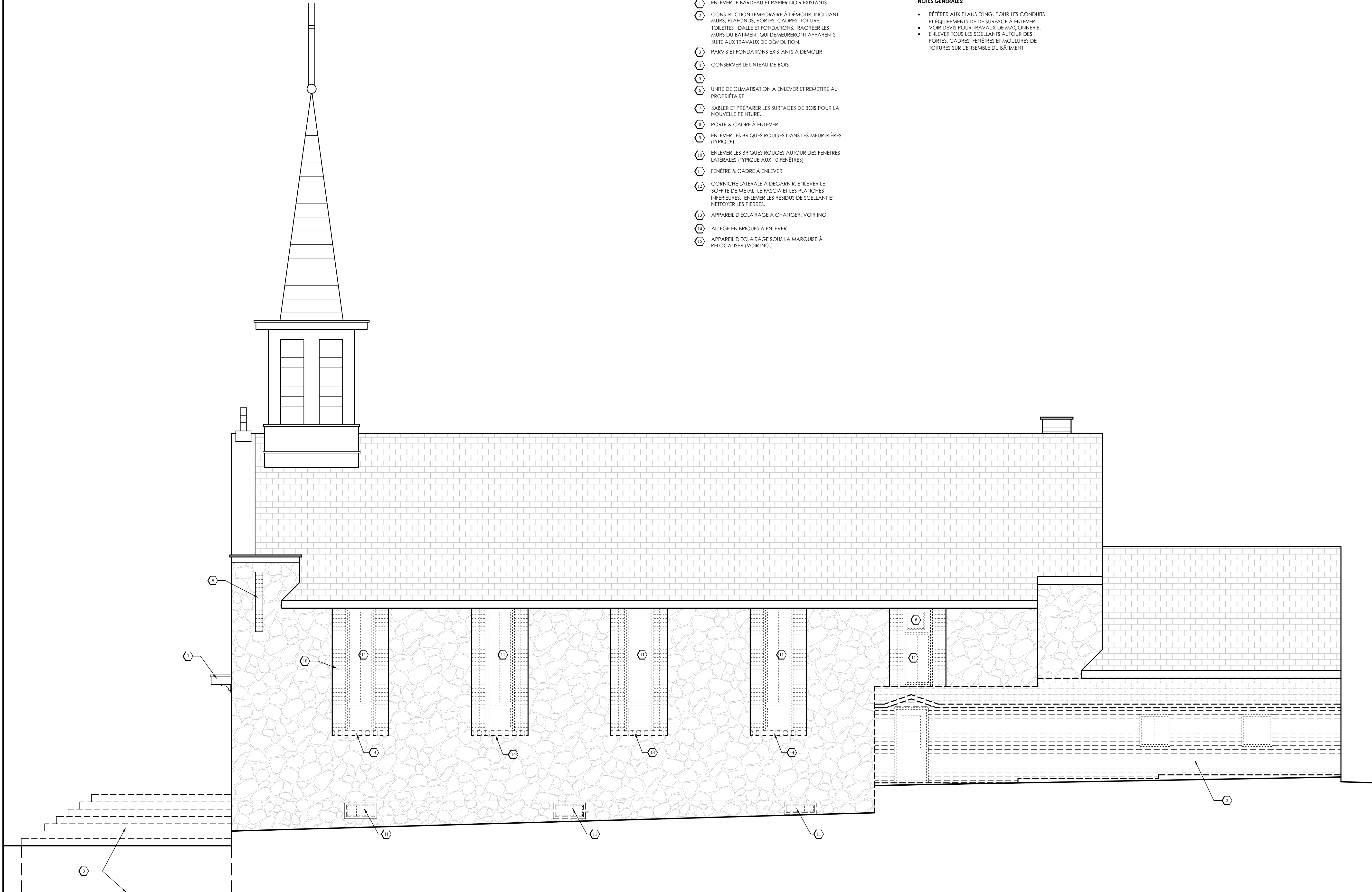
1 A5 ÉLÉVATION LATÉRALE DROITE EXISTANT & DÉMOLITION
